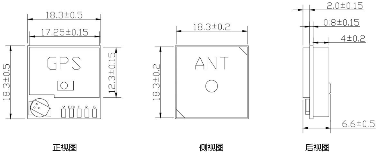
图 2：产品规格图
